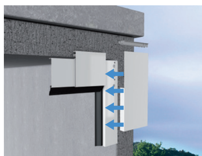
Universal-Blendenlösung, Außenansicht
