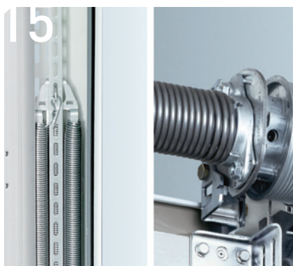
15 Senkrechte Zugfeder für Garagen-Sektionaltore
